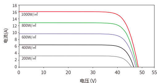
电流-电压曲线 66HL4M-(V) 615W
